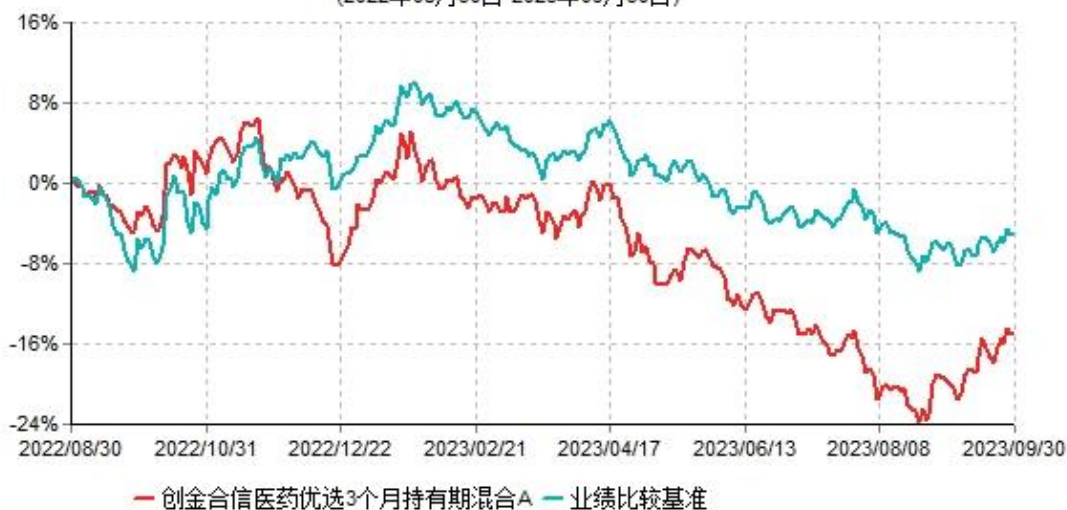
创金合信医药优选3个月持有期混合A累计净值增长率与业绩比较基准收益率历史走势对比图 (2022年08月30日-2023年09月30日)
