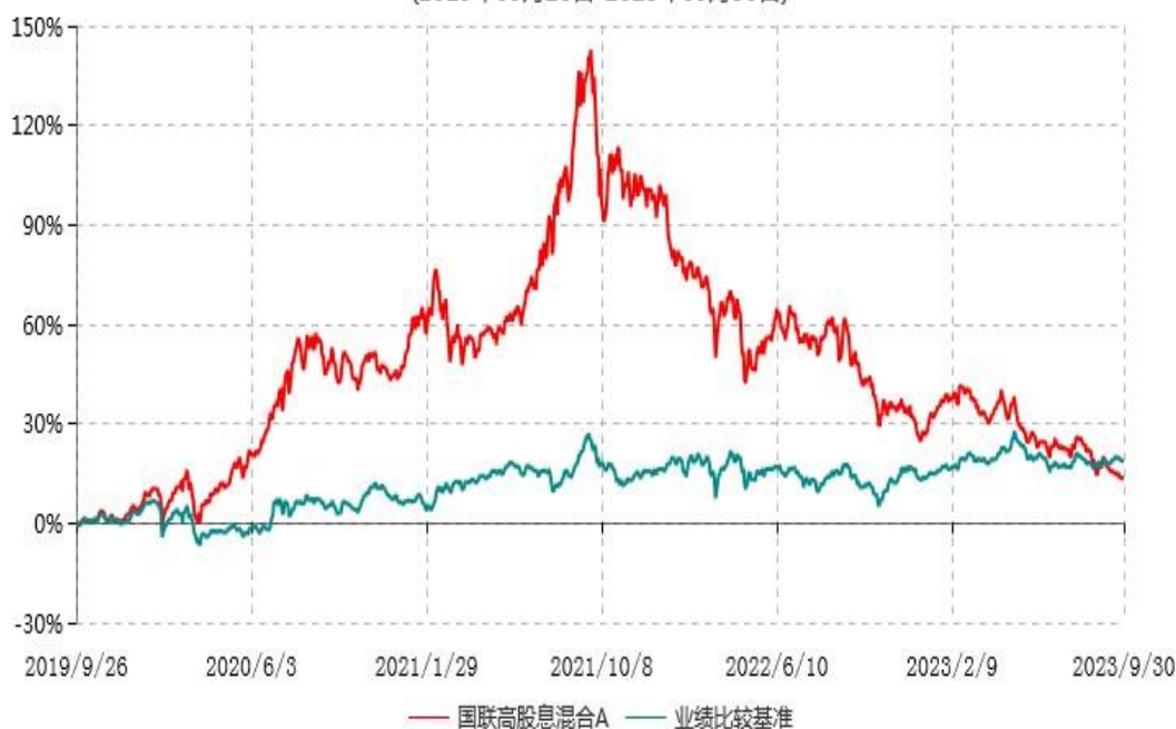
国联高股息混合A累计净值增长率与业绩比较基准收益率历史走势对比图
