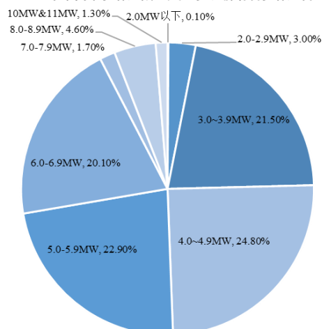
2022年不同单机容量陆上风电机组新增装机容量占比
