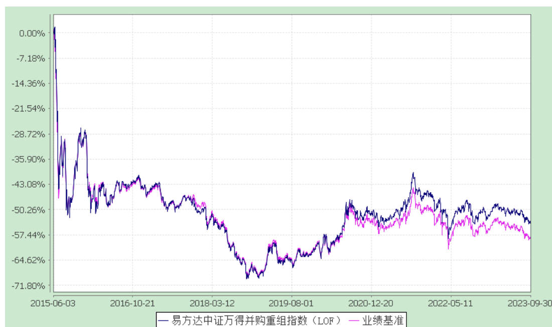
易方达中证万得并购重组指数证券投资基金（LOF） 累计净值增长率与业绩比较基准收益率的历史走势对比图 (2015 年 6 月 3 日至 2023 年 9 月 30 日)
