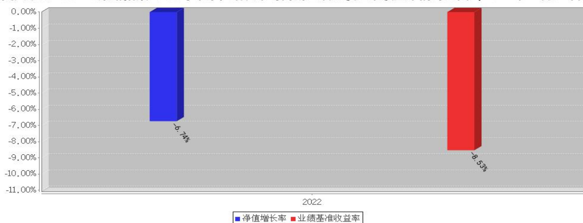
英大中证 ESG120 策略指数 A 基金每年净值增长率与同期业绩比较基准收益率的对比图（2022 年 12 月 31 日）
