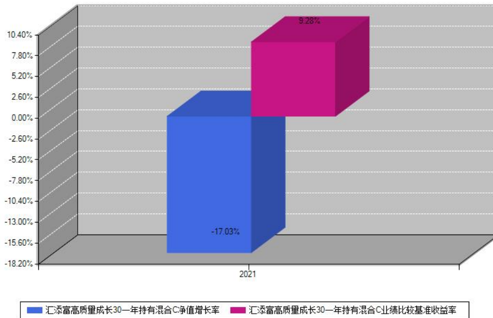
汇添富高质量成长30一年持有混合C每年净值增长率与同期业绩基准收益率对比图
