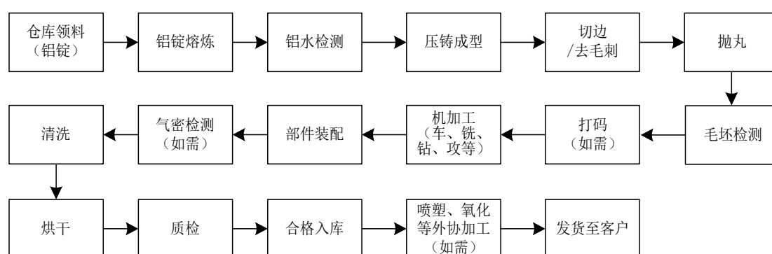
图：生产工序流程
