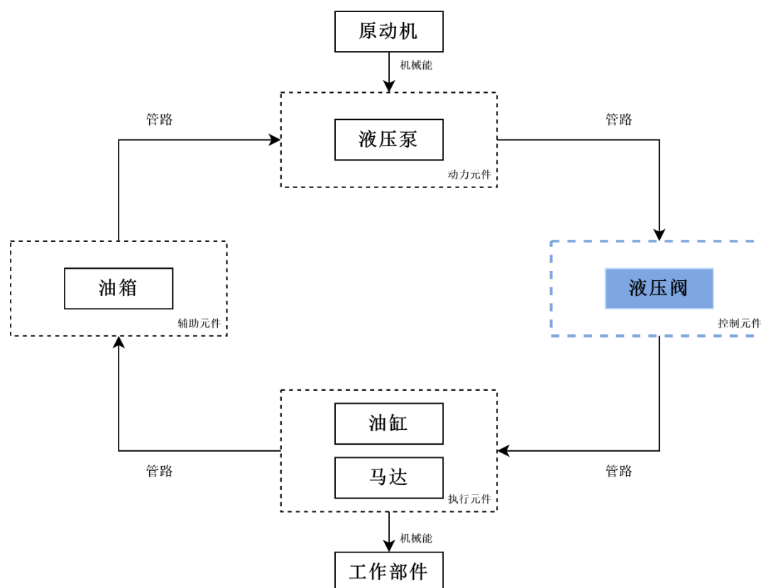
液压系统工作原理图
