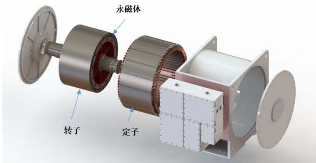
永磁同步电机分解示意图
