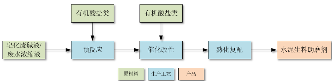
甘油醚生产工艺流程：
