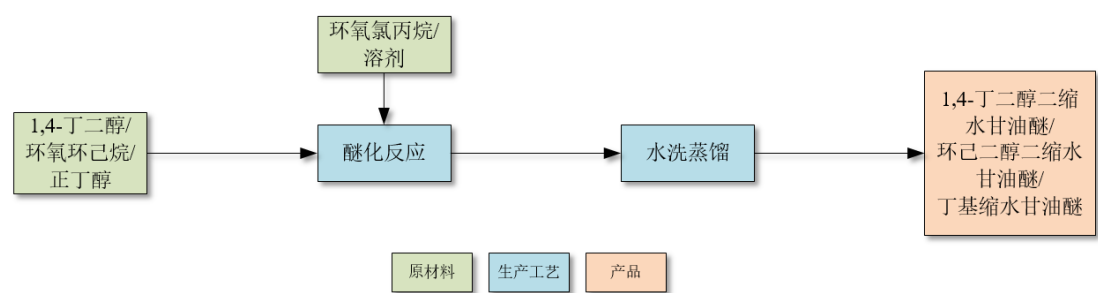
环己二醇单甲醚生产工艺流程：
