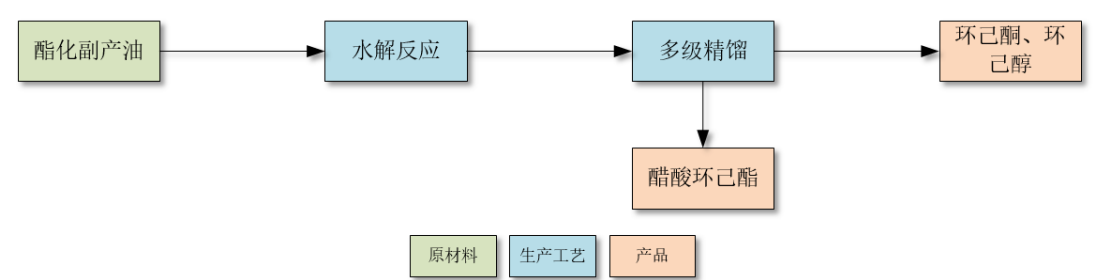
皂化液废碱液综合利用工艺流程：
