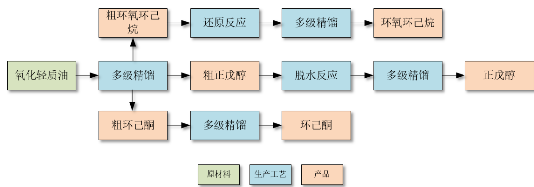
酯化副产油综合利用工艺流程：
