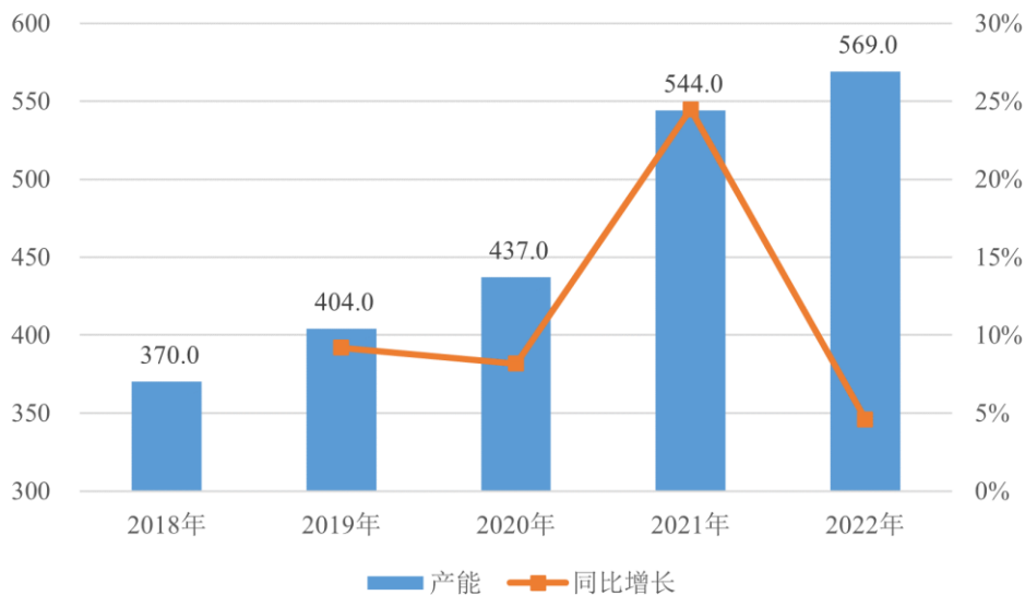
2018–2022 年中国己内酰胺产能及增长率（单位：万吨）
