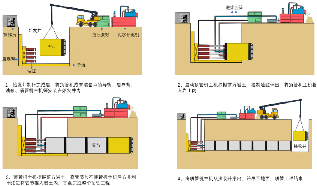
机械顶管法示意图
