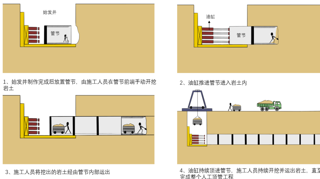
人工顶管法示意图
