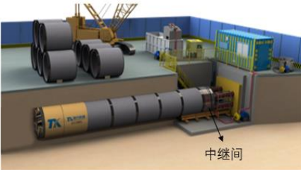
5、启动主机，利用油缸将第一节管节推入岩土内，并重复以上步骤，直至完成整个顶管工程。如长距离顶进，油缸推力不足时，则加入中继间提供中继顶力
