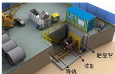
1、始发井制作完成后，将导轨、后靠背、油缸安装在始发井内
