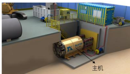
2、将主机放入始发井的导轨上
