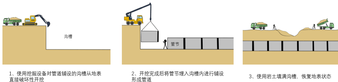
明挖法示意图
