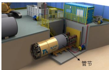
4、收回油缸，放入第一节管节
