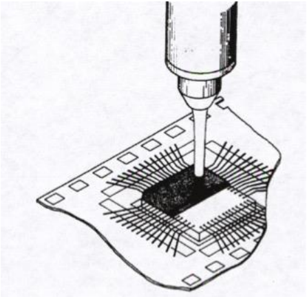
图：TAB密封
