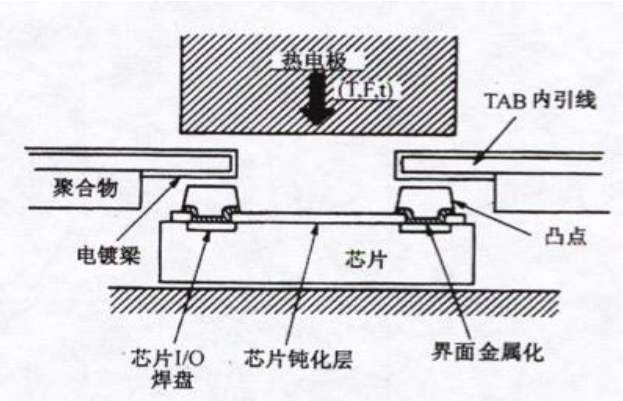
图：TAB 内引线键合
