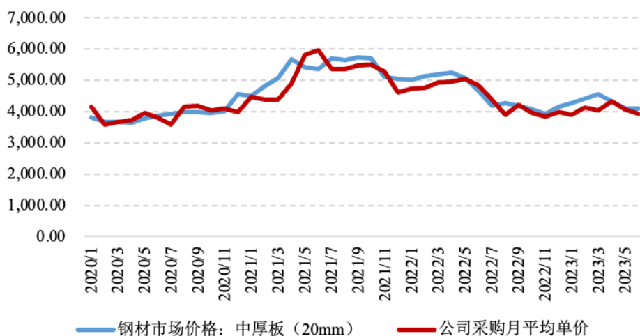
公司钢材价格与市场价格（元/吨）
