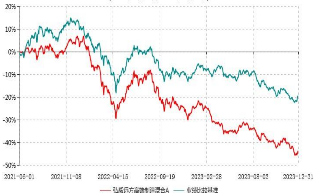
弘毅远方高端制造混合A累计净值增长率与业绩比较基准收益率历史走势对比图
