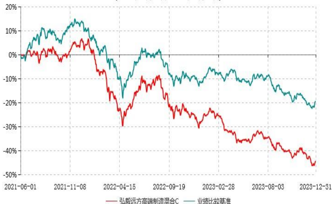
弘毅远方高端制造混合C累计净值增长率与业绩比较基准收益率历史走势对比图 (2021年06月01日-2023年12月31日)
