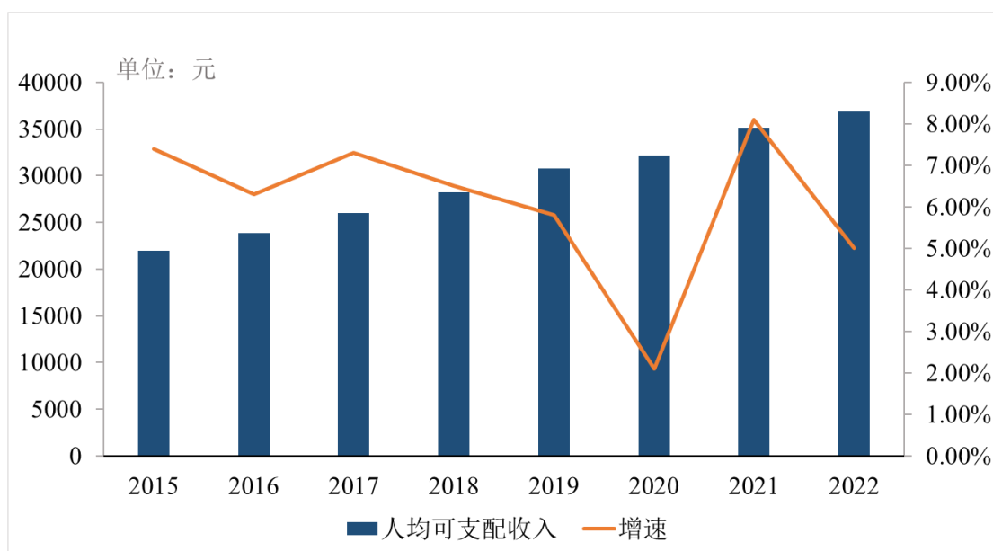
居民人均可支配收入
