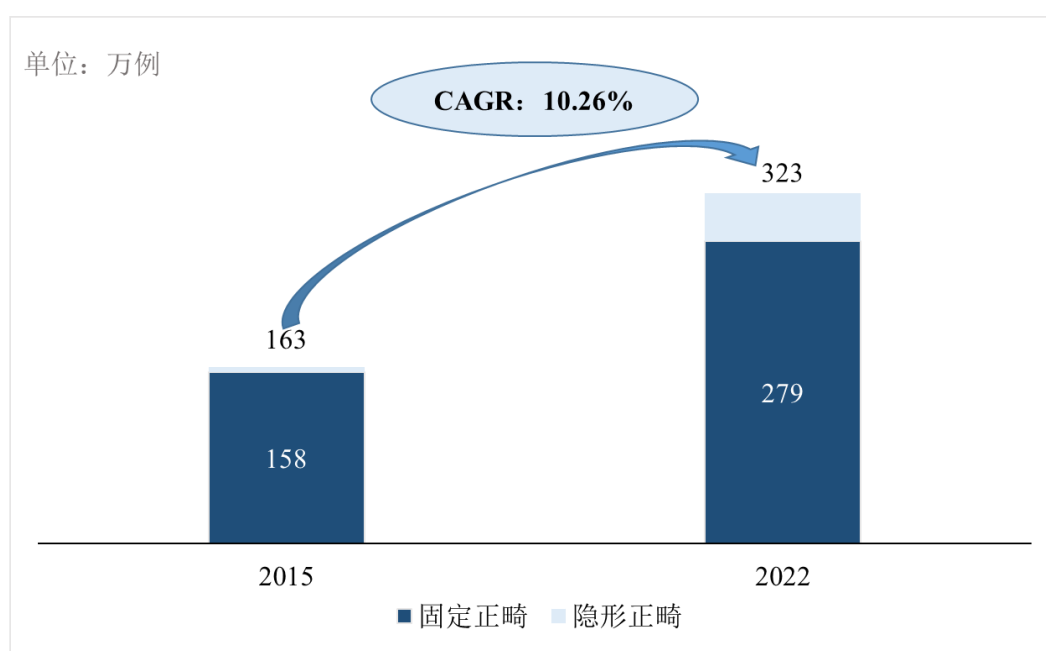
中国正畸案例数
