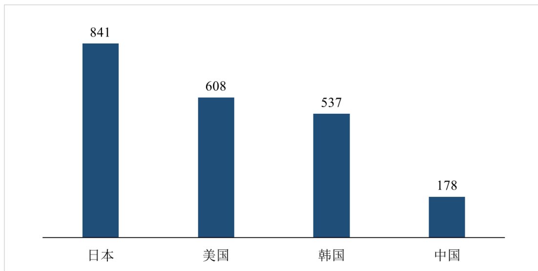
每百万人口牙医数量（2021 年）
