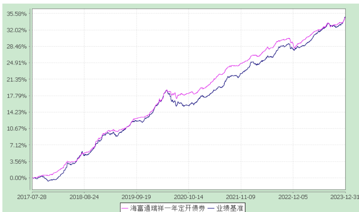
海富通瑞祥一年定期开放债券型证券投资基金 份额累计净值增长率与业绩比较基准收益率历史走势对比图 (2017 年 7 月 28 日至 2023 年 12 月 31 日)
