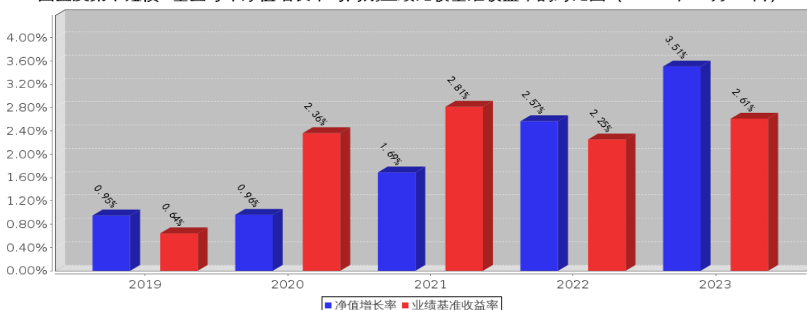
国金及第中短债A基金每年净值增长率与同期业绩比较基准收益率的对比图（2023年12月31日）
