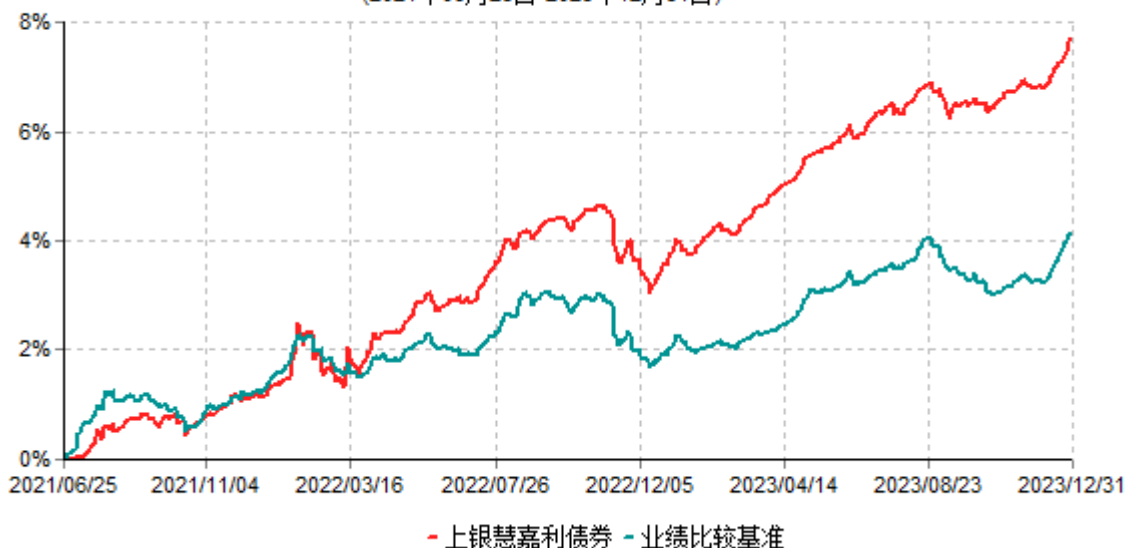
上银慧嘉利债券型证券投资基金累计净值增长率与业绩比较基准收益率历史走势对比图 (2021年06月25日-2023年12月31日)
