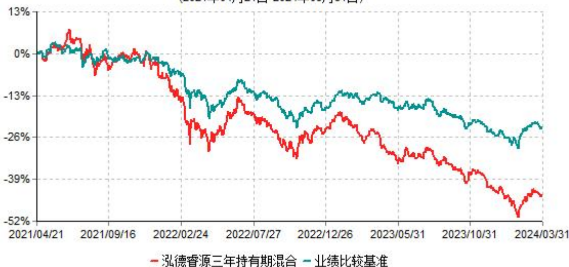
泓德睿源三年持有期灵活配置混合型证券投资基金累计净值增长率与业绩比较基准收益率历史走势对比图 (2021年04月21日-2024年03月31日)
