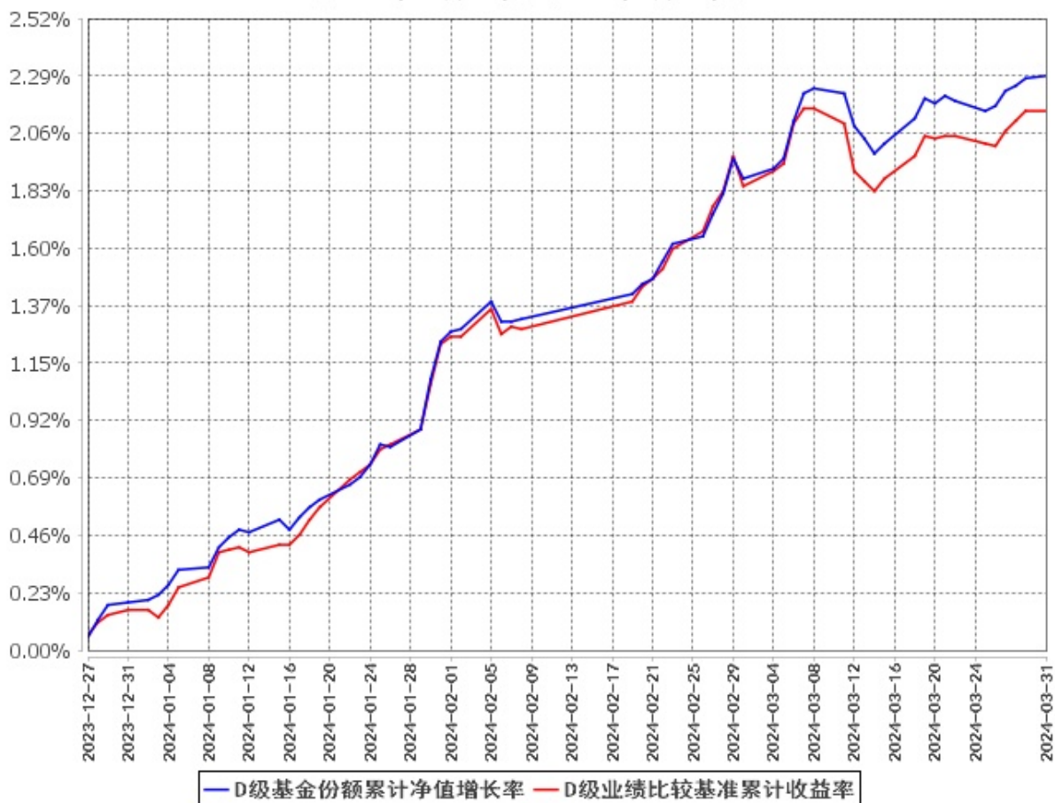
D级基金份额累计净值增长率与同期业绩比较基准收益率的历史走势对比图 (2023年12月27日至2024年3月31日)
