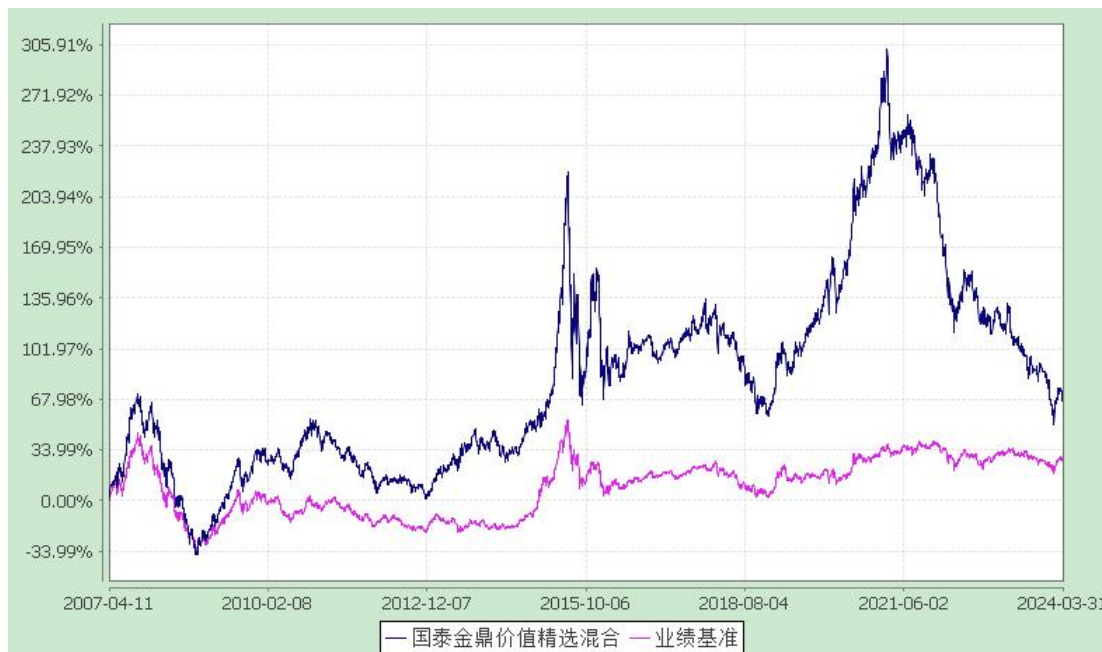
国泰金鼎价值精选混合型证券投资基金 累计净值增长率与业绩比较基准收益率历史走势对比图 (2007 年 4 月 11 日至 2024 年 3 月 31 日)
