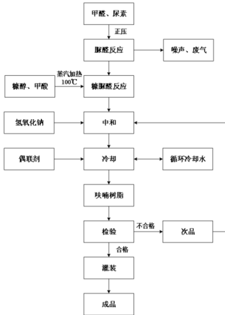
(1) 呋喃树脂工艺路线图
