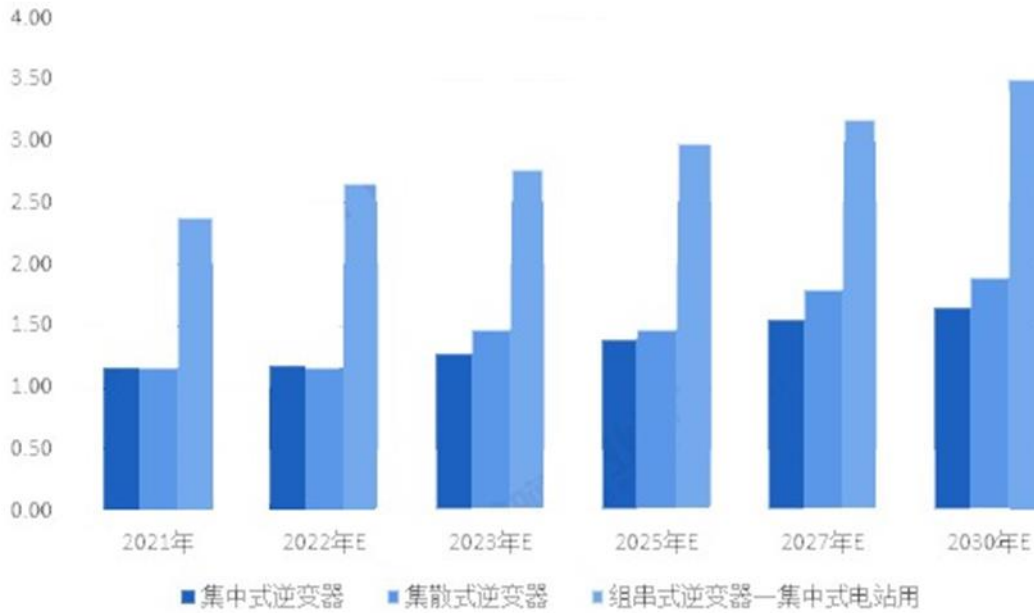
2021-2030年中国光伏逆变器功率密度变化趋势(单位: kW/kg)
