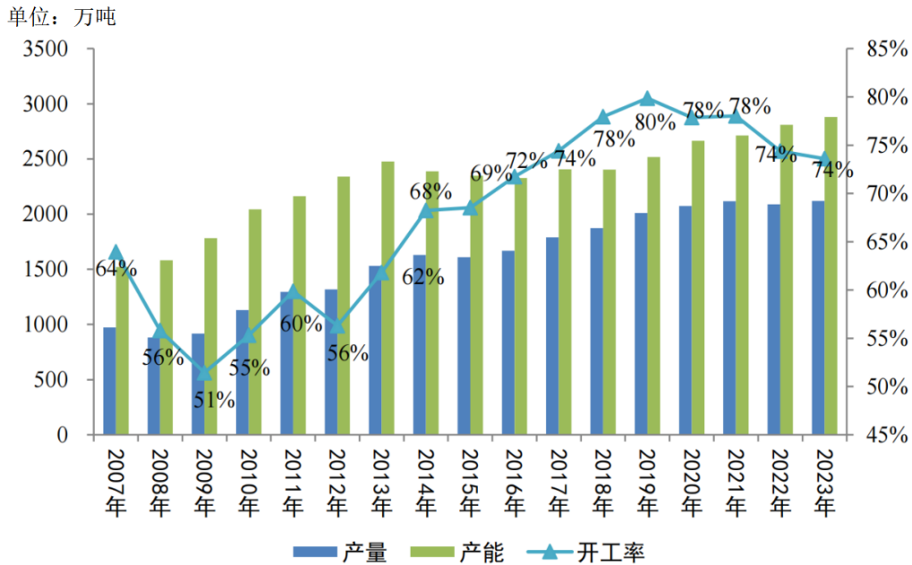
2007-2023年我国PVC产能产量及开工率变化趋势
