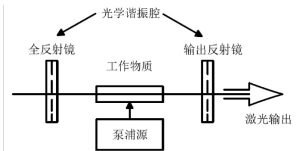
图表 1 激光器结构图
