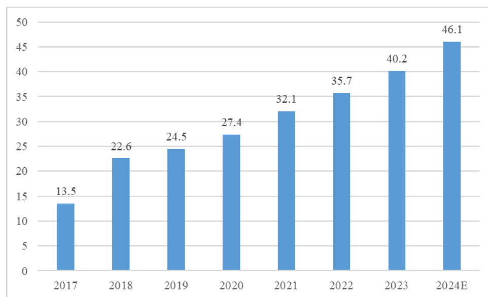
图表 19 2017-2024E 年中国超快激光器市场规模（含进口,单位：亿元）
