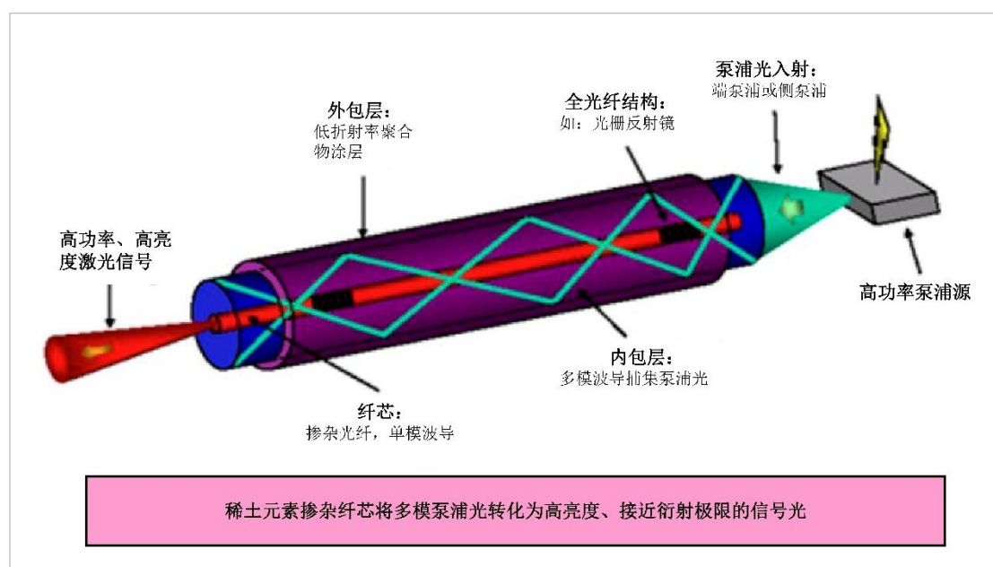
图表 10 光纤激光器结构示意图
