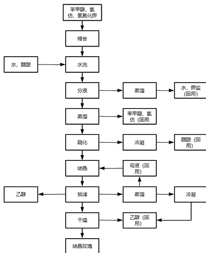
②结晶玫瑰的生产流程图
