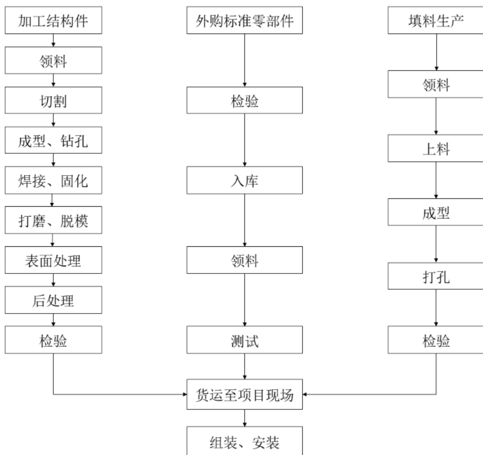
2) 空气能水—水热泵机组工艺流程图
