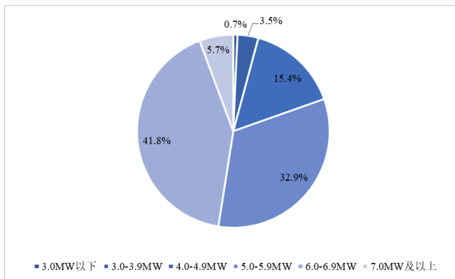
2023 年我国陆上不同单机容量风电机组新增装机容量占比
