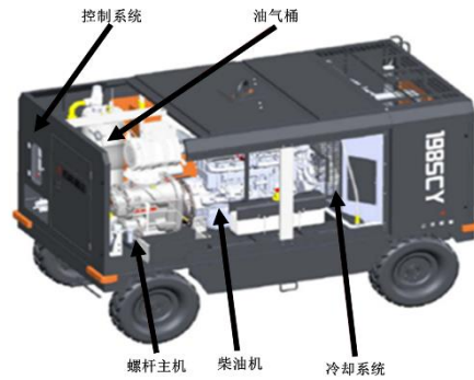
柴油机驱动螺杆机
