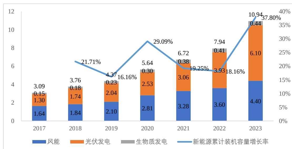
2017 年-2023 年中国新能源发电结构（亿千瓦）
