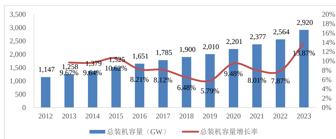
2012 年-2023 年中国发电装机容量（GW）
