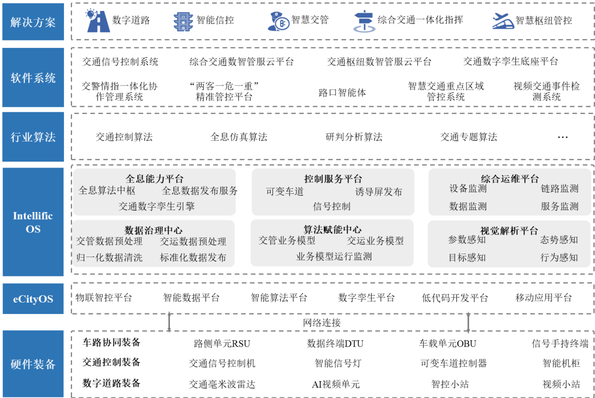
图：城市交通业务架构
