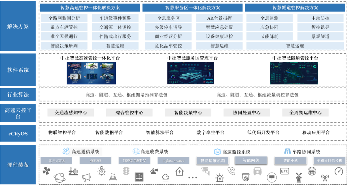
图：公路交通业务架构
