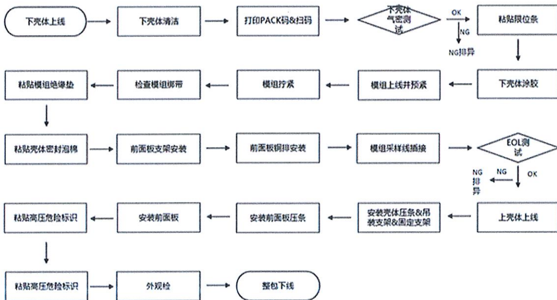
Pack 工艺流程图
