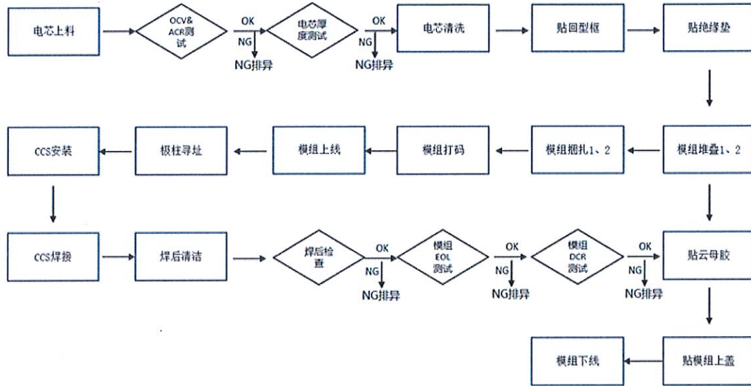
模组工艺流程图
