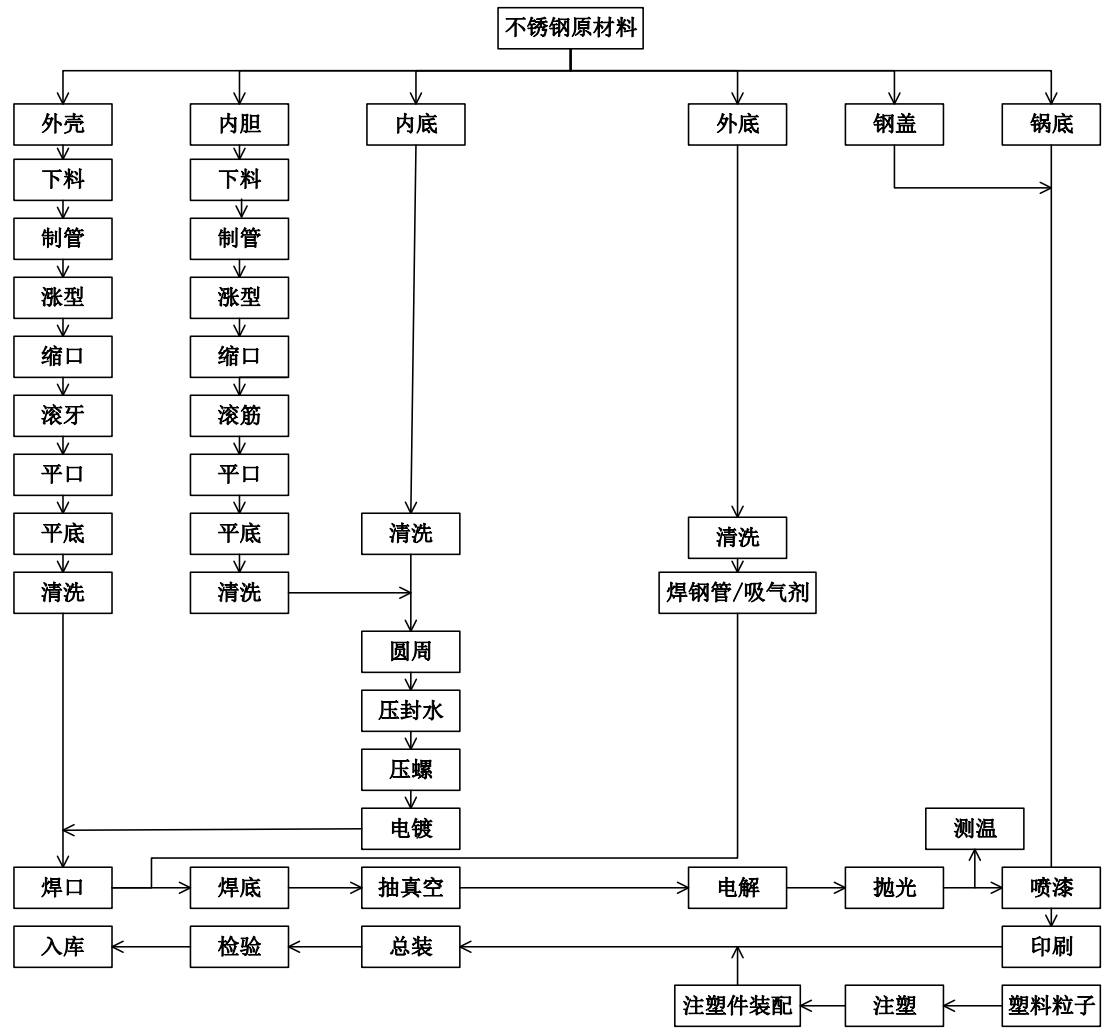
(2) 公司保温箱生产工艺流程图
