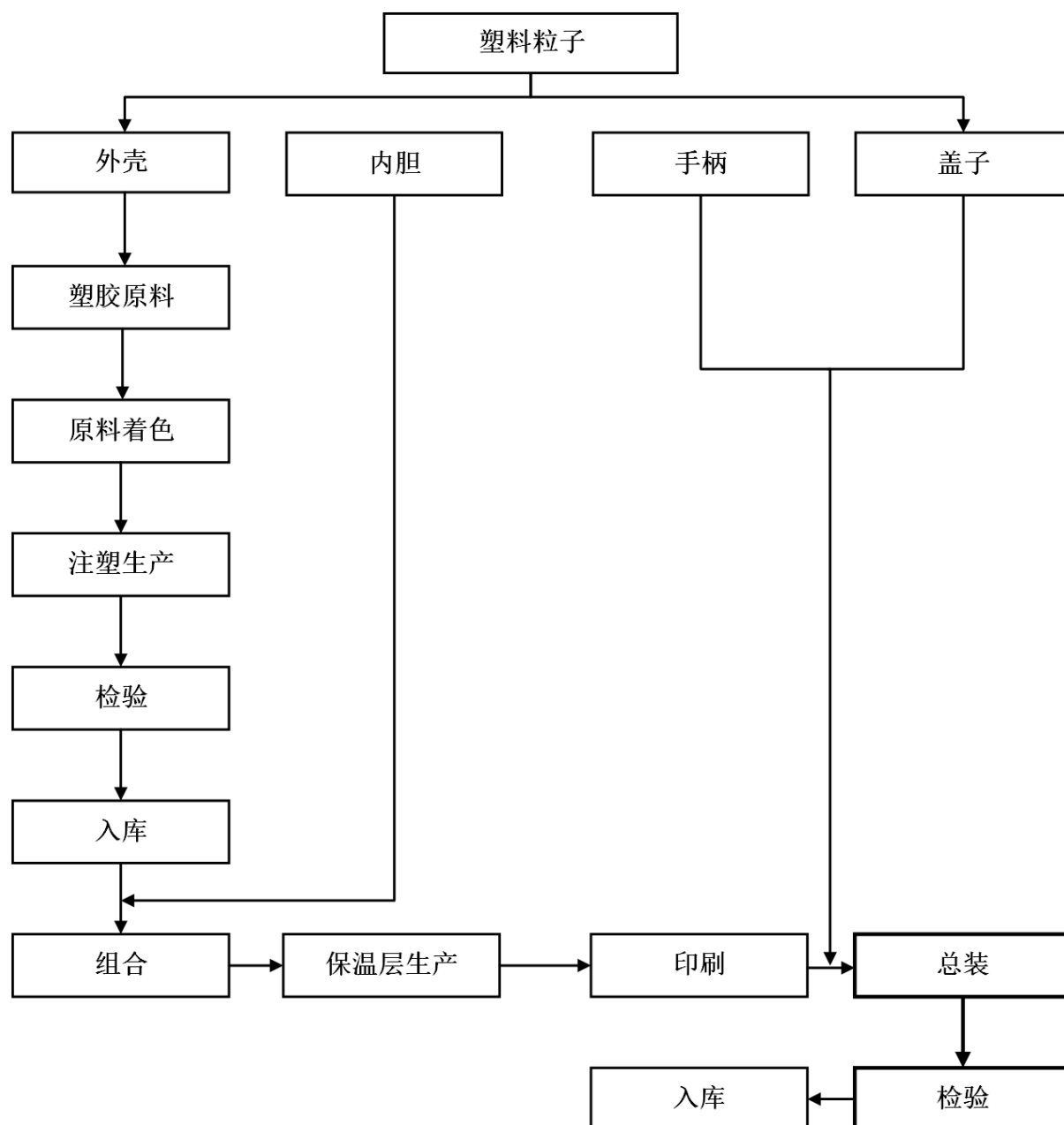
(3) 公司玻璃杯生产工艺流程图
