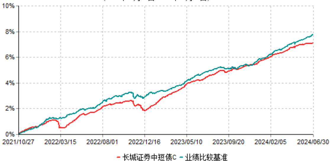
长城证券中短债C累计净值增长率与业绩比较基准收益率历史走势对比图 (2021年10月27日-2024年06月30日)
