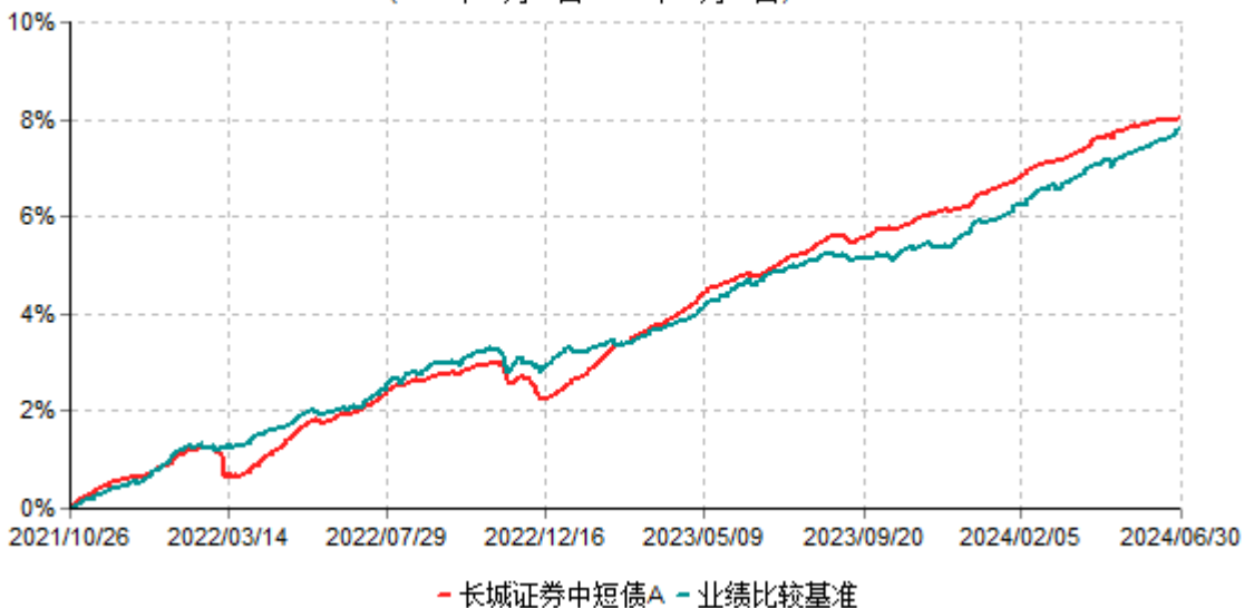
长城证券中短债A累计净值增长率与业绩比较基准收益率历史走势对比图 (2021年10月26日-2024年06月30日)
