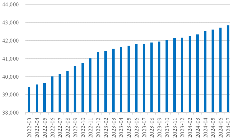
我国水力发电累计装机容量（万千瓦）
