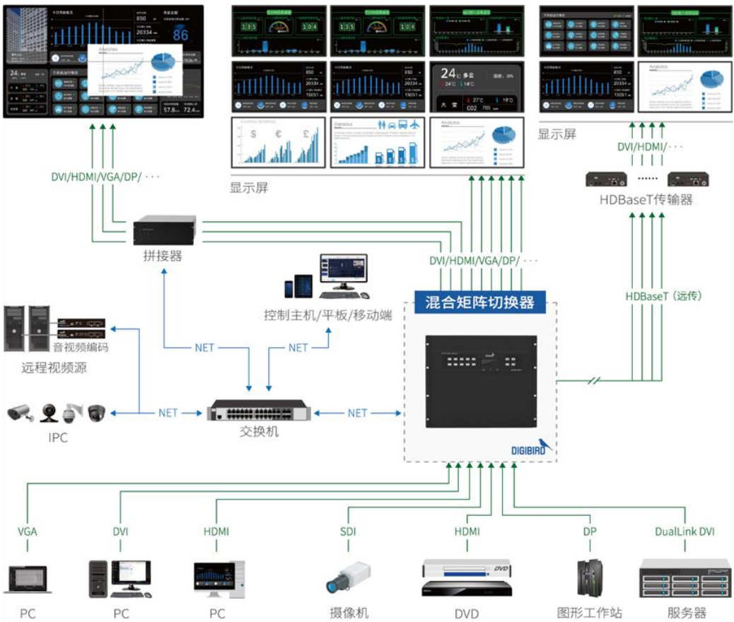
混合矩阵切换器应用拓扑图
