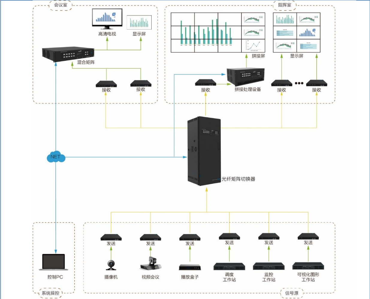
光纤矩阵切换器应用拓扑图
