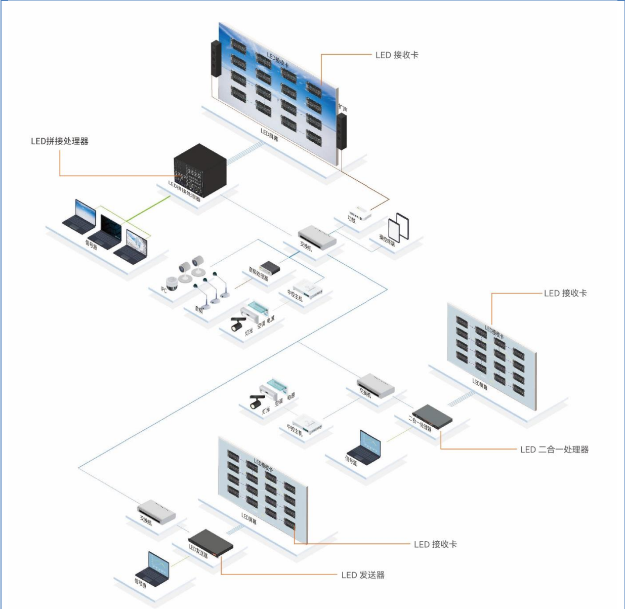
LED 显示控制设备应用拓扑图
