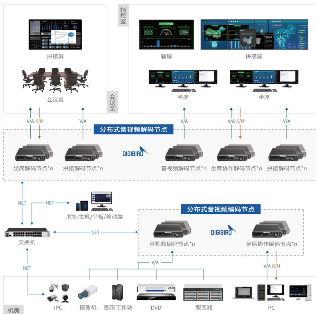
分布式音视频处理设备应用拓扑图
