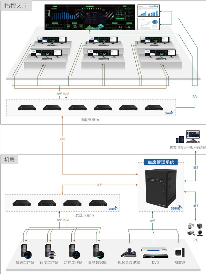
坐席管理设备应用拓扑图
