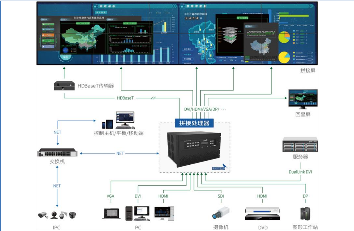
大屏拼接设备应用拓扑图
