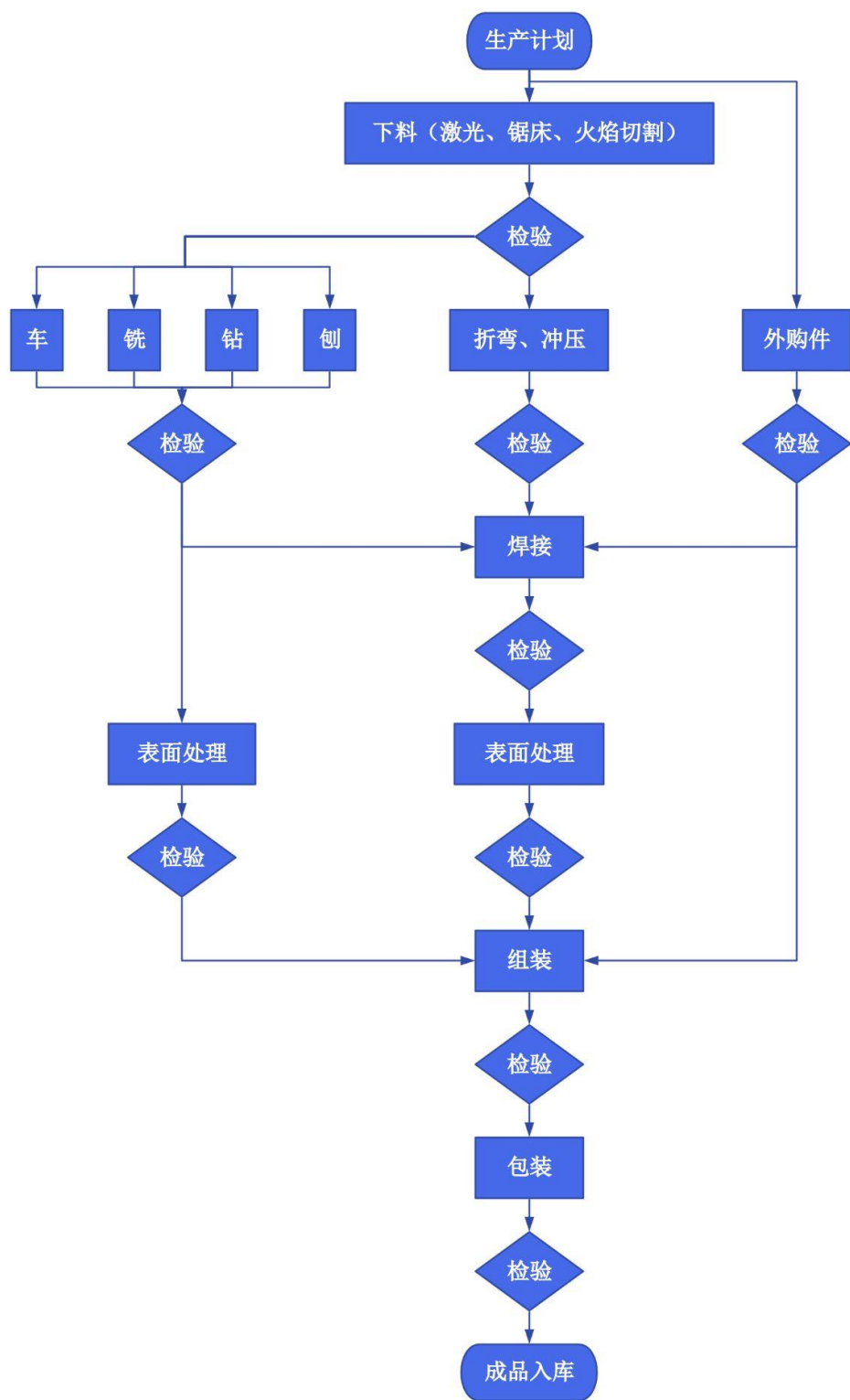
② 公司拆胎机和平衡机工艺流程
