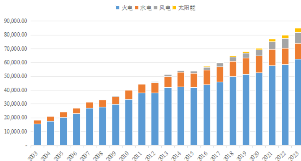
全国发电量结构（单位：亿千瓦时）
