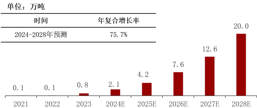
中国钠电正极材料出货量，2021-2028 年预测
