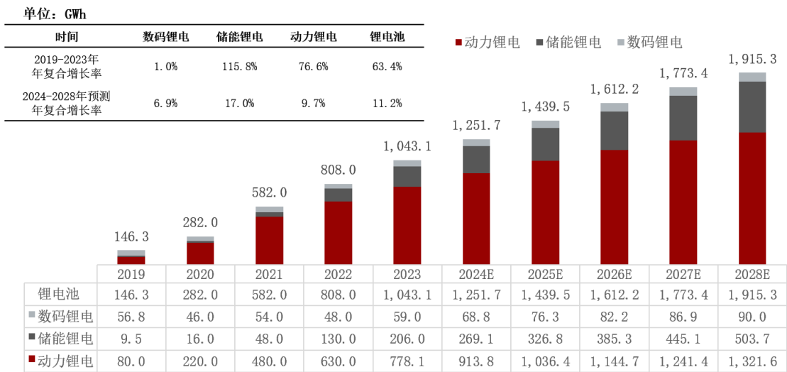
中国锂离子电池出货量，2019–2028 年预测
