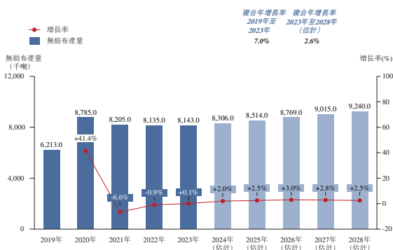
無紡布的產量（中國）， 2019年至2028年（估計）
