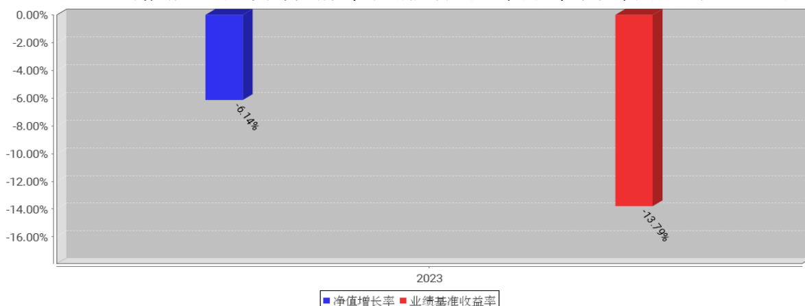
工银中证1000指数增强A基金每年净值增长率与同期业绩比较基准收益率的对比图（2023年12月31日）
