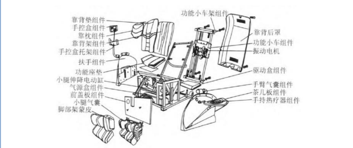
图：按摩椅结构图
