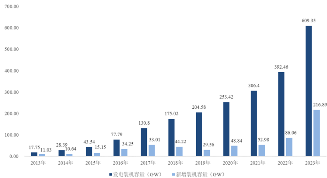
图：2013 年-2023 年我国光伏发电装机容量情况
