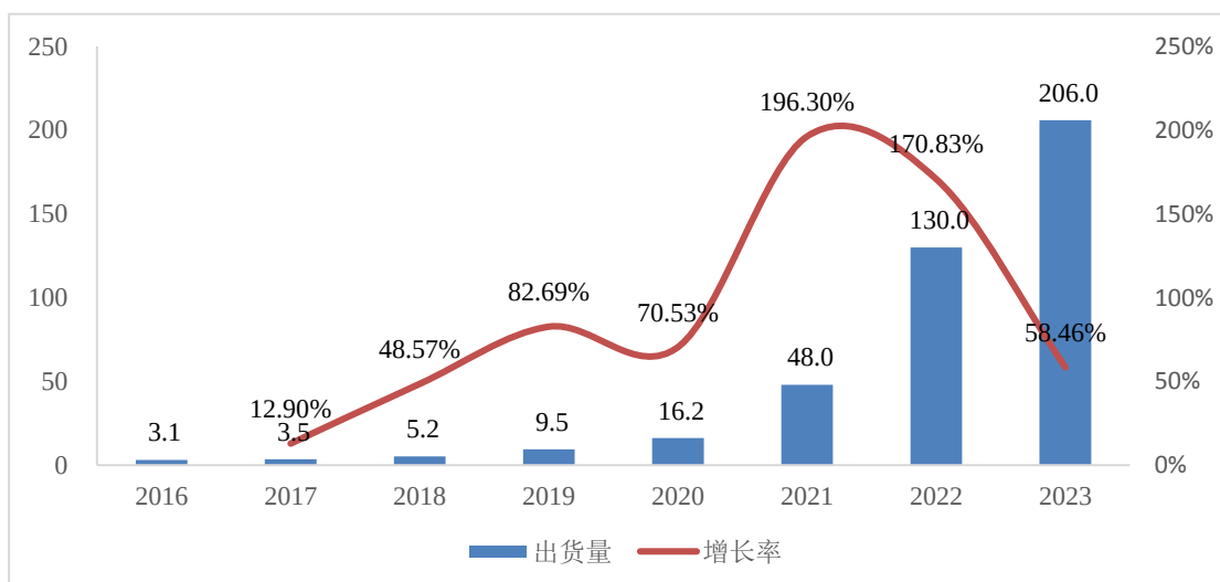
2016 年-2023 年中国储能电池出货量（GWh）
