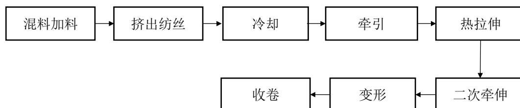
图：弯丝主要生产工艺流程
