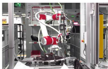
车灯锁螺丝
