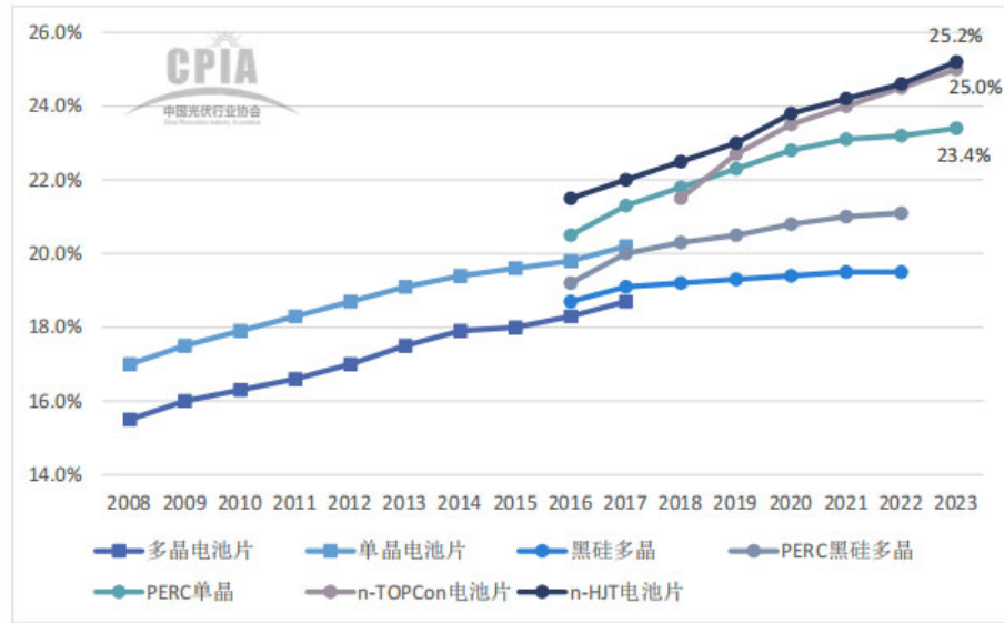
图：2008-2023 年我国电池片量产转换效率发展趋势
