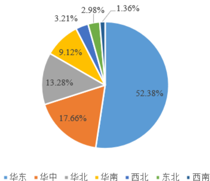
2024年6月30日分布式光伏电站累计装机容量区域分布
