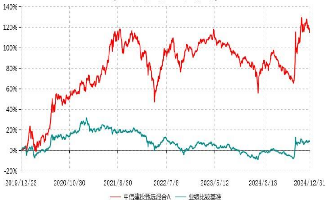
中信建投甄选混合A累计净值增长率与业绩比较基准收益率历史走势对比图 (2019年12月23日-2024年12月31日)
