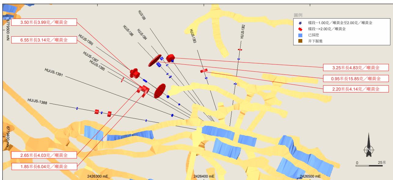
圖4－Arpola-5平面圖。
