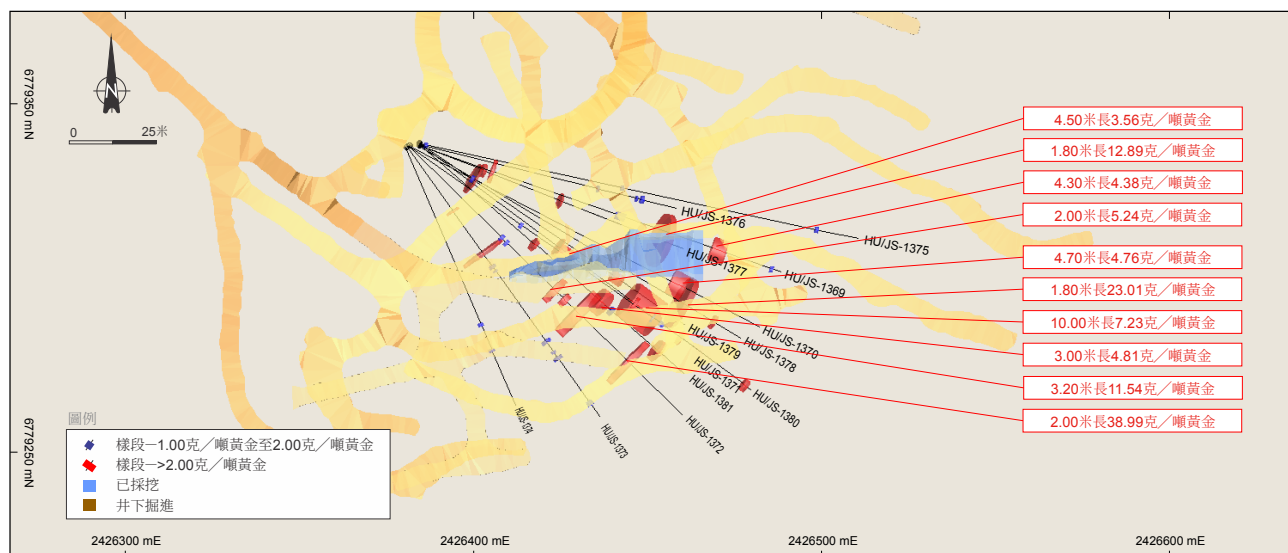
圖2—Arpola-4平面圖。
